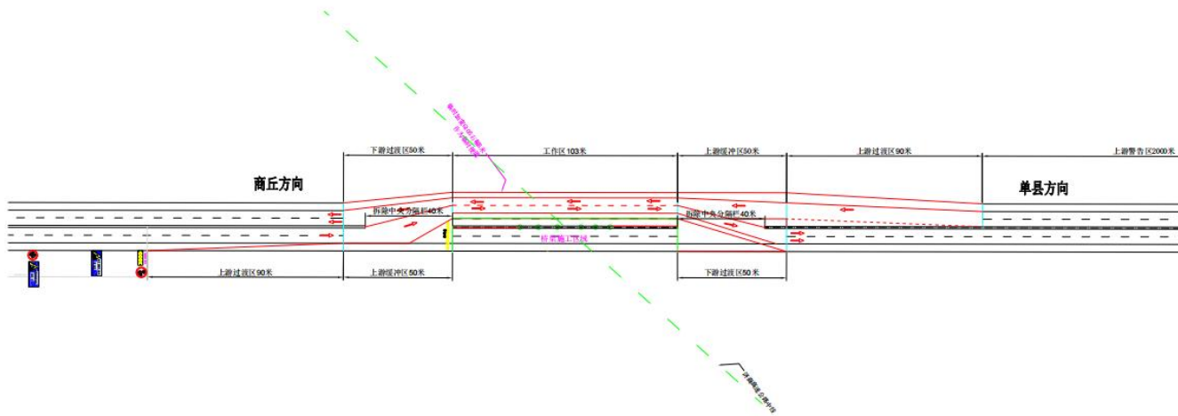
第一阶段、第二阶段导改方式示意图
